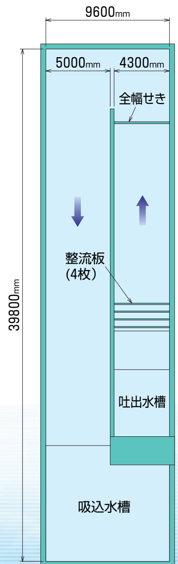
大型試験水槽全景
